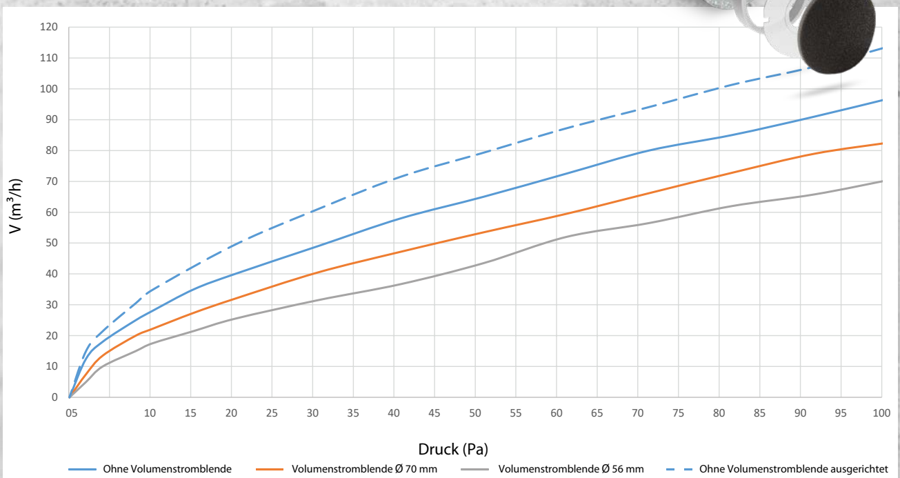
Druck-Volumenstrom-Kennlinie ALD-SV
